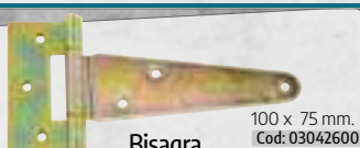
Bisagra bicromatada 507
